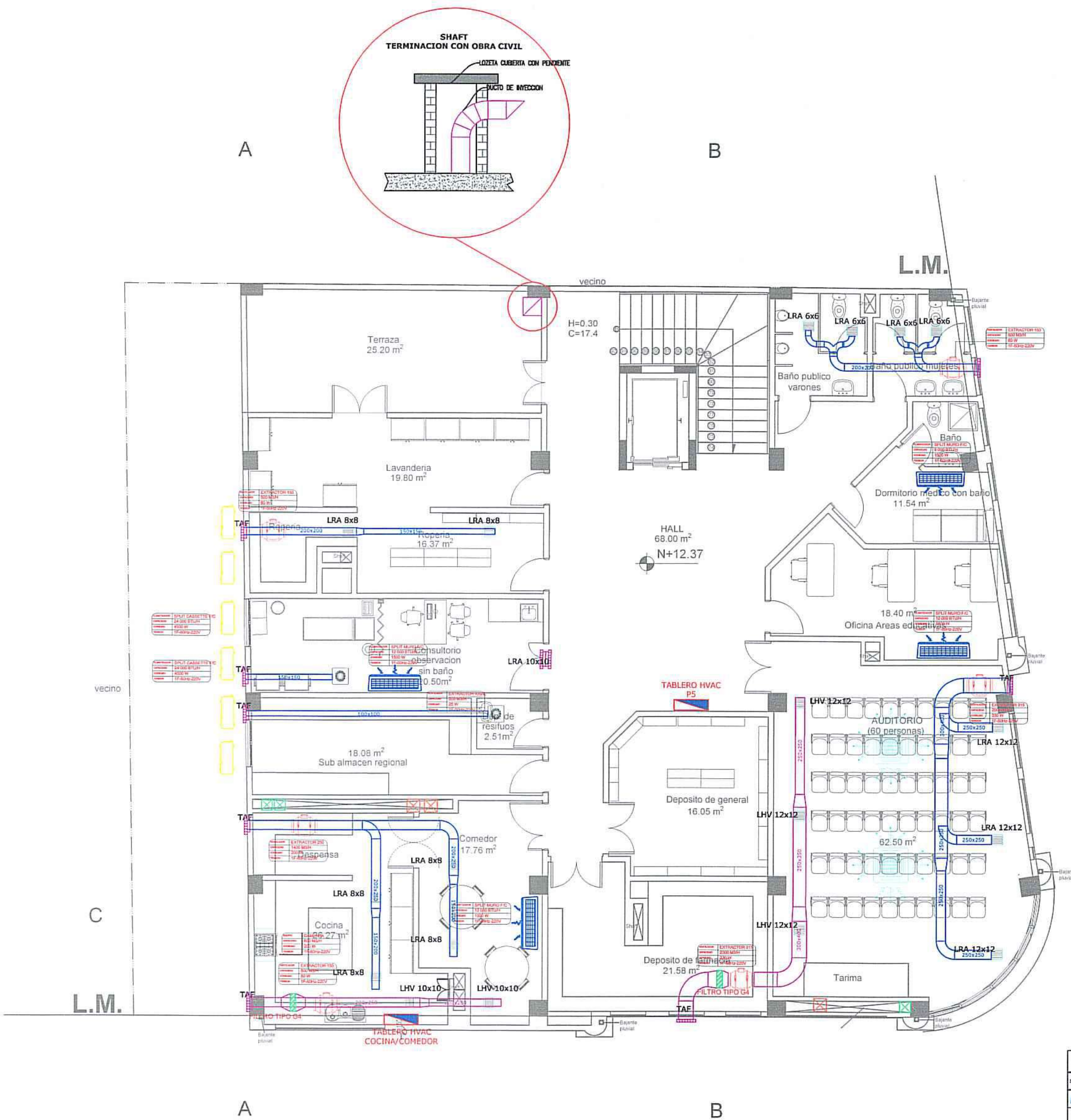
PLANTA Nivel 05
